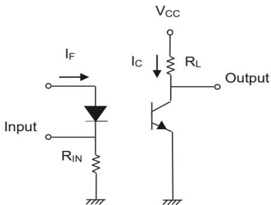
图例 11-开关时间测试电路图
